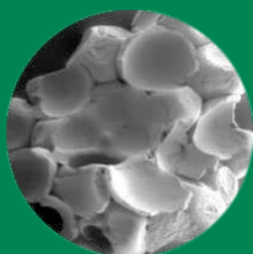
MACRO-POROSIDAD 200-500 \mu\text{m}
