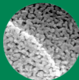
NANOPOROSIDAD 40-80 nm
